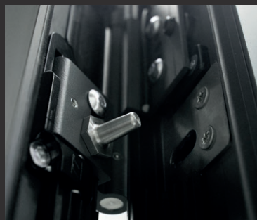
Антизломні болти - це додаткове устаткування, яке покращує антизломні характеристики дверей. Вони встановлюються з боку петель на дверному полотні та на коробці. Залежно від необхідного ступеню безпеки можна застосовувати різну кількість наборів для одного полотна.
